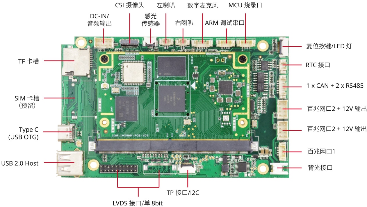
接口示意图：
